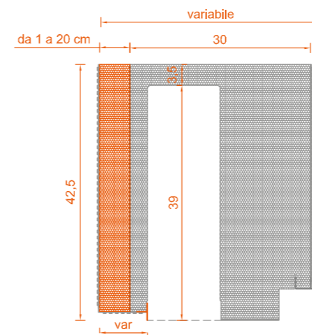
ECL1 SU MISURA con spalla maggiorata esterna/interna
