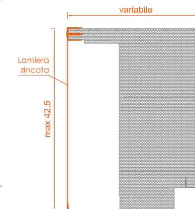
ECL2 SU MISURA con lamiera esterna zincata
