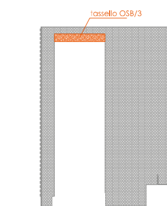
ECL6 SU MISURA con tassello in OSB/03 per fissaggio frangisole NON autoportante
