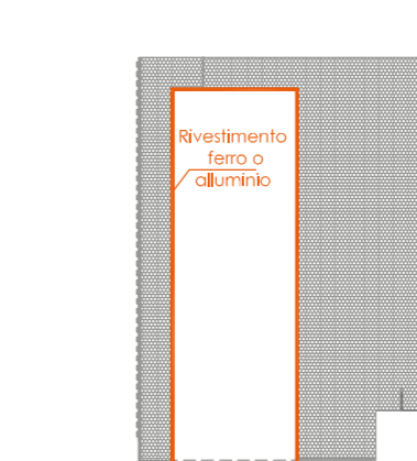
ECL5 SU MISURA rivestimento interno in ferro o alluminio zincato
