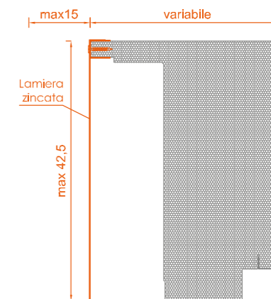
ECL3 SU MISURA con lamiera zincata con porta cappotto
